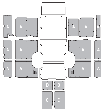
Fahrzeugtyp - Model L4 H3
